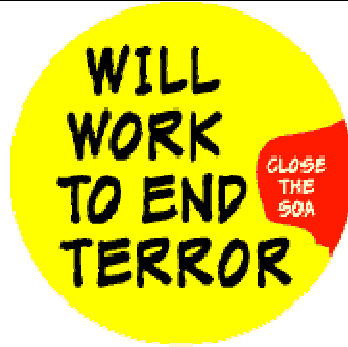
SOA-WWTETerror
