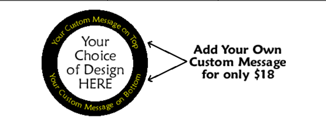
SOA-WWFP
