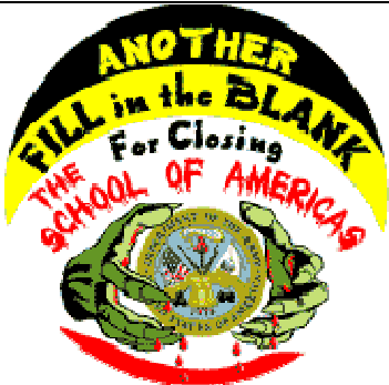
SOA_A_FC
